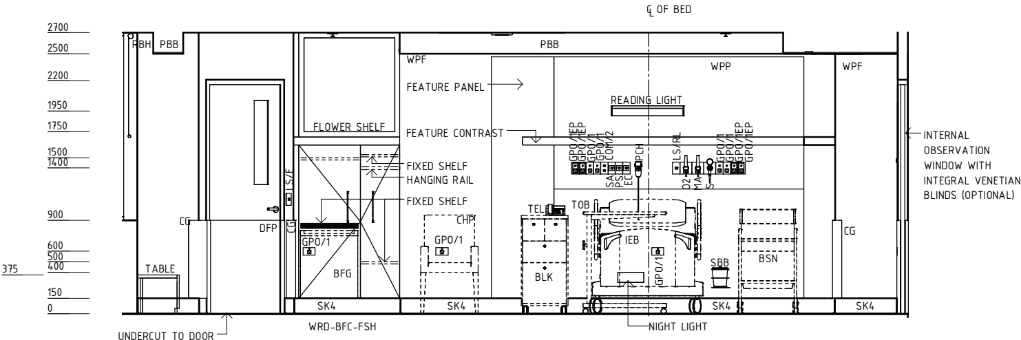
ELEVATION 2
