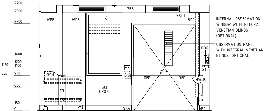
ELEVATION 3
