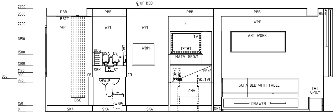
ELEVATION 4
